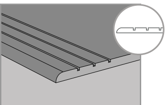
“INCISIONI ANTISCIVOLO” ANTISLIP ENGRAVING
