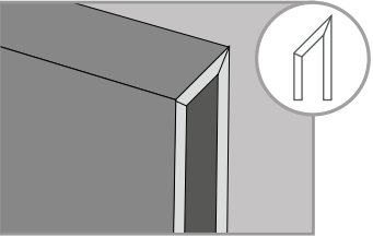
“DOPPIA ELLE SLOPE” SLOPE DOUBLE L-SHAPE
