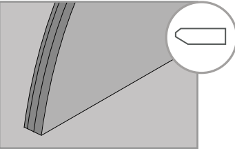
“CHAMFER” Bisello Maggiorato + ripresa della costa fatta a mano + taglio jolly a 30° Shimmed Bevel + handmade edge finish + 30° miter
