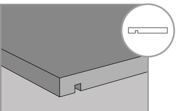
“SCANALATURA ROMPIGOCCIA” DRIP GROOVE FOR SILL
