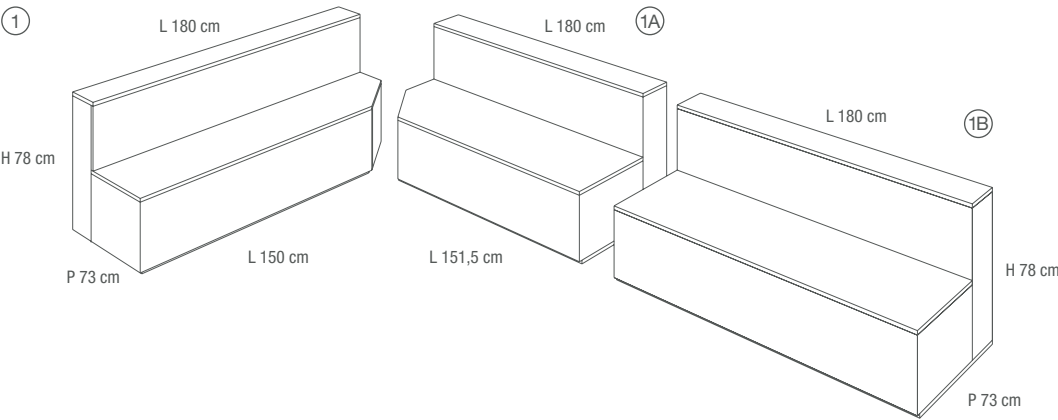
PANCA 2.0 LAVORAZIONE A “ELLE” CON “RIPRESA DELLA COSTA” BENCH IN 20mm L-SHAPE AND EDGE FINISH
