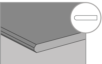
“DOPPIO BISELLO MAGGIORATO” DOUBLE SHIMMED BEVEL
